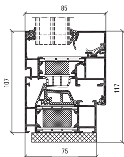
Profilmått fönster, skala 1:4
