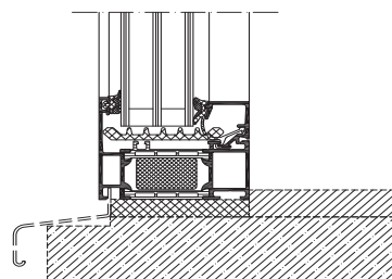
Anslutningsprincip fast fönster, skala 1:4
