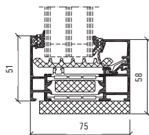
Profilmått fast fönster, skala 1:4
