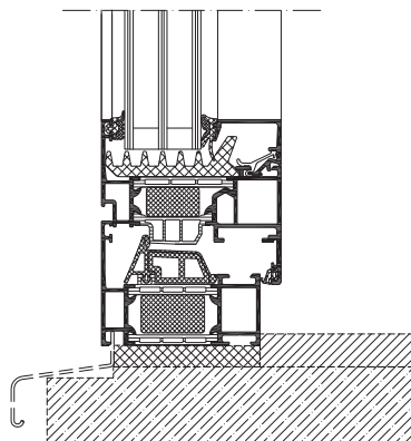
Anslutningsprincip öppningsbart fönster, skala 1:4
