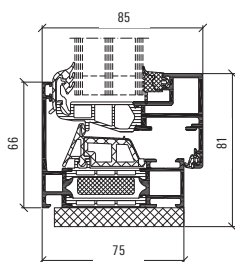
Profilmått, skala 1:4
