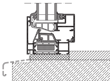
Anslutningsprincip öppningsbart fönster, skala 1:4
