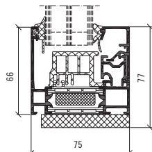
Profilmått, skala 1:4
