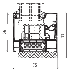
Profilmått fast fönster skala, 1:4
