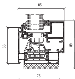
Profilmått öppningsbart fönster, skala 1:4
