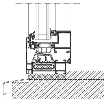
Anslutningsprincip öppningsbart fönster, skala 1:4
