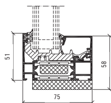
Profilmått fast fönster, skala 1:4
