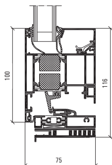
Profilmått fönster skala, 1:4
