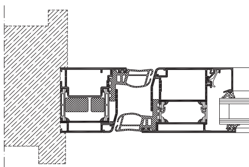
Anslutningsprincip för klämfri bakkant, skala 1:4
